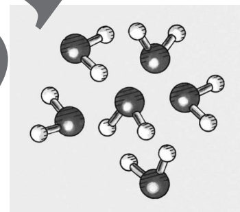
Abb. 4: Wassermolekül
