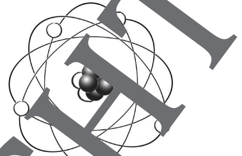
Abb. 3: Atommodell von Bohr
