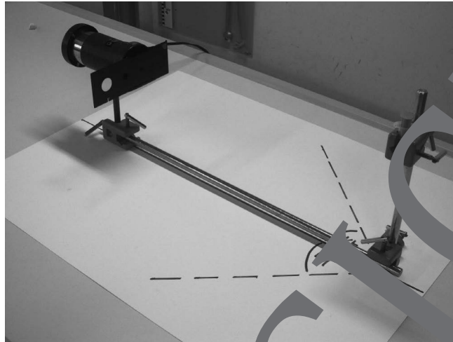
Versuchsanordnung zum Schülerversuch „Entstehende Wassertropfen“; links oben: Experimentierneuchte mit Lochblende, zentral: Blatt mit beidseitig eingezeichneten Peillinien zum Unterlegen, rechts: Stativ mit Spritz-
