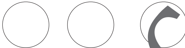
Kochsalz
